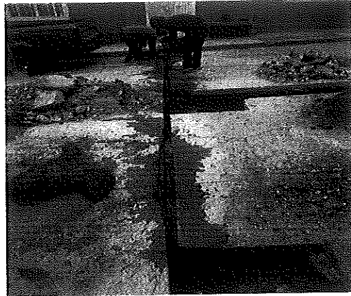
Reparación toma en Corregidora
